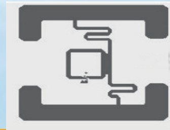
天线示意图
